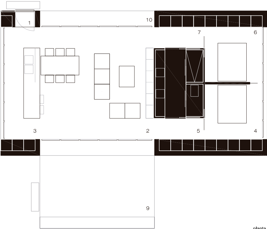
planta baja e_1/100
